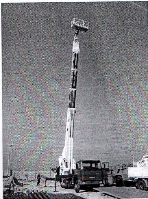
Slika 1a i 1b. Hidraulična polužna kamionska dizalica sa platformom
